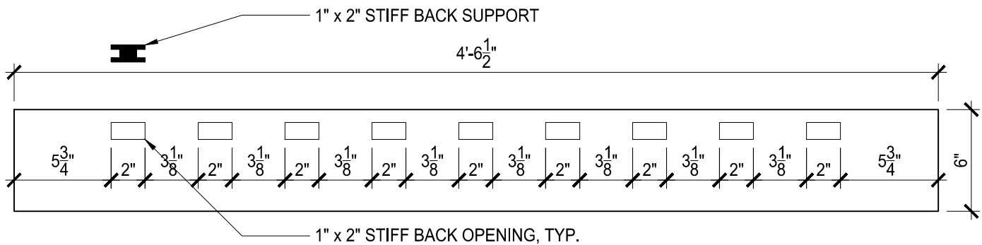
ELEVATION SIDE D:
